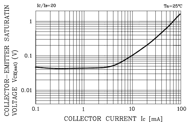
Fig. 2 V_{CE(SAT)} - I_C
