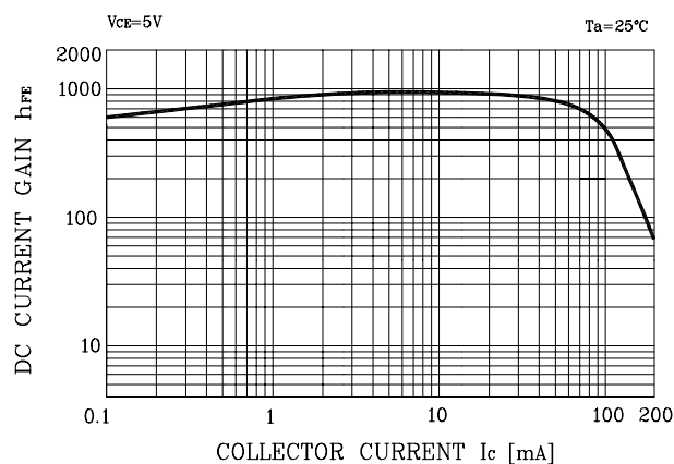
Fig. 1 h_{FE} - I_C
