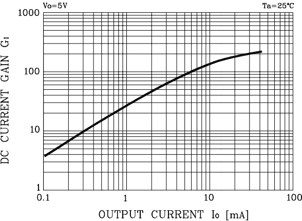
Fig. 3 G_I - I_O
