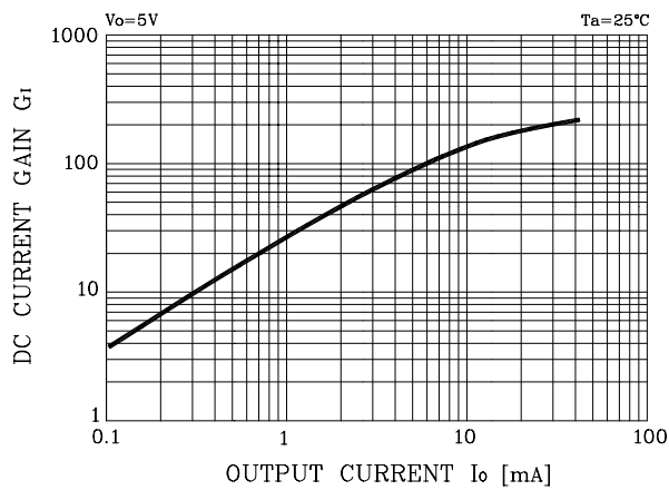
Fig. 3 G_I - I_O
