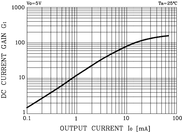
Fig. 3 G_I - I_O
