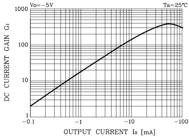
Fig. 3 G_I - I_O
