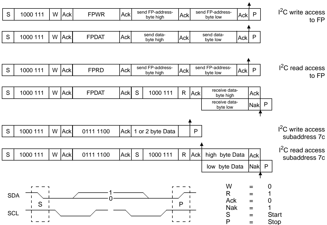
Fig. 3–1: I 2 C-bus protocols
