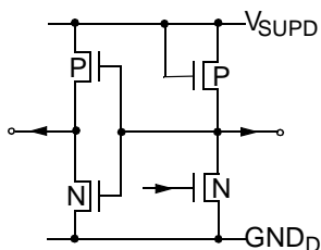
Fig. 4-5: Input/Output pin FPDAT
