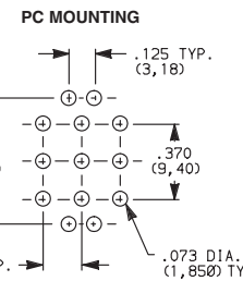
E301J1_BE2 3PDT
