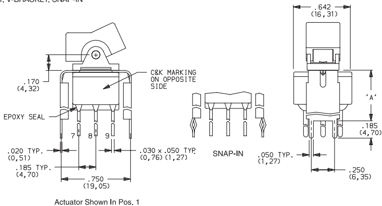
E301J1_BE2 3PDT
