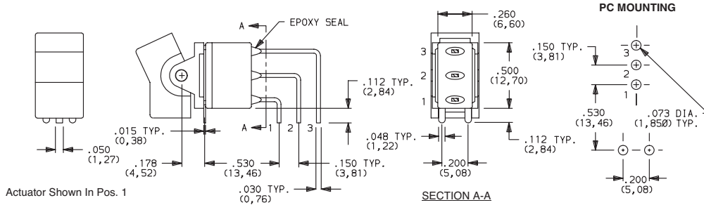
E101J1V5BE2 Vertical Actuation SPDT
