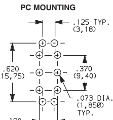
E201J1_BE2 DPDT
