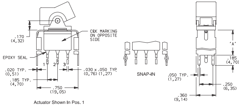
E101J1_BE2 SPDT
