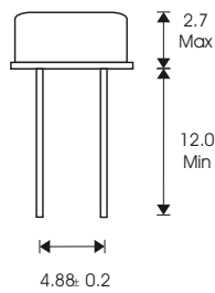
HC-49/SS
