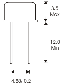
HC-49/S
