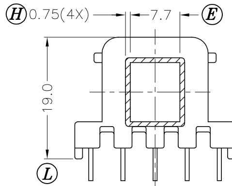
SEC.A-A
