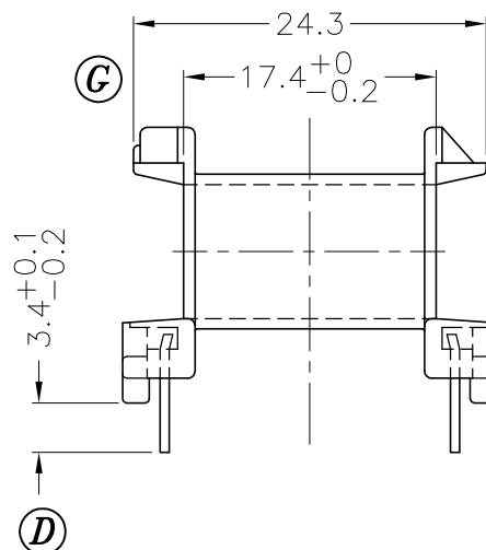
SEC.A-A
