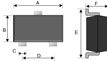
SOT-23
