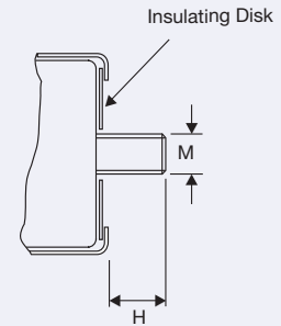
ALS37 Stud Mounting
