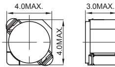
DIMENSIONS (mm) 外形寸法図
