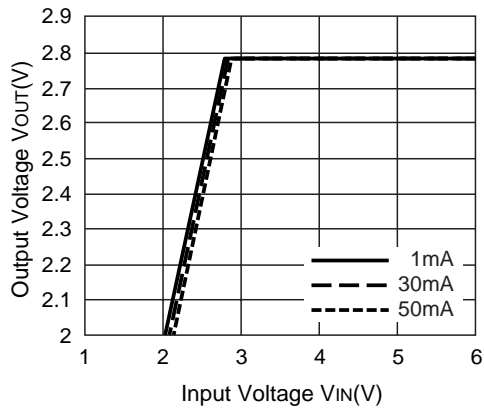
2.8V (VR1)
