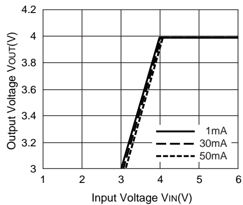
4.0V (VR1)
