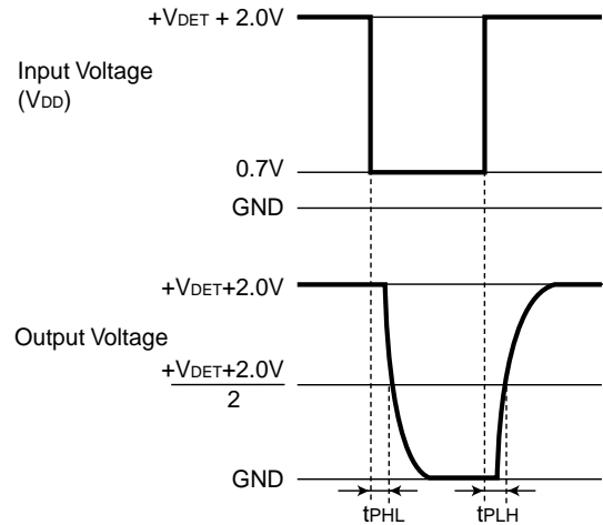
CMOS Output
