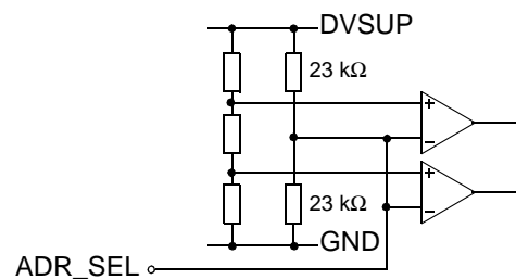
Fig. 4-17: Input Pin: ADR_SEL
