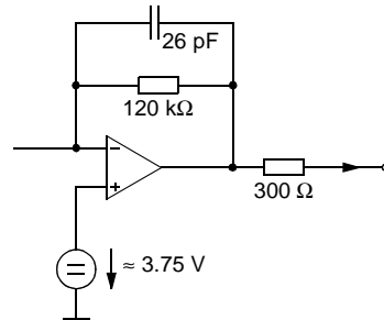
Fig. 4-22: Output Pins: SC_2_OUT_R/L, SC_1_OUT_R/L
