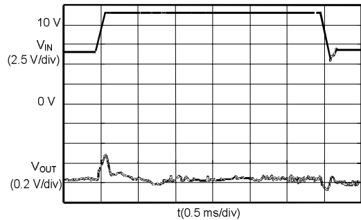
S-8520/1E33MC ( I_{OUT} :10 mA)
