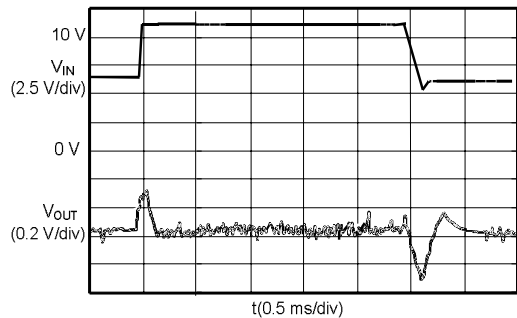
S-8520/1E33MC ( I_{OUT} :500 mA)
