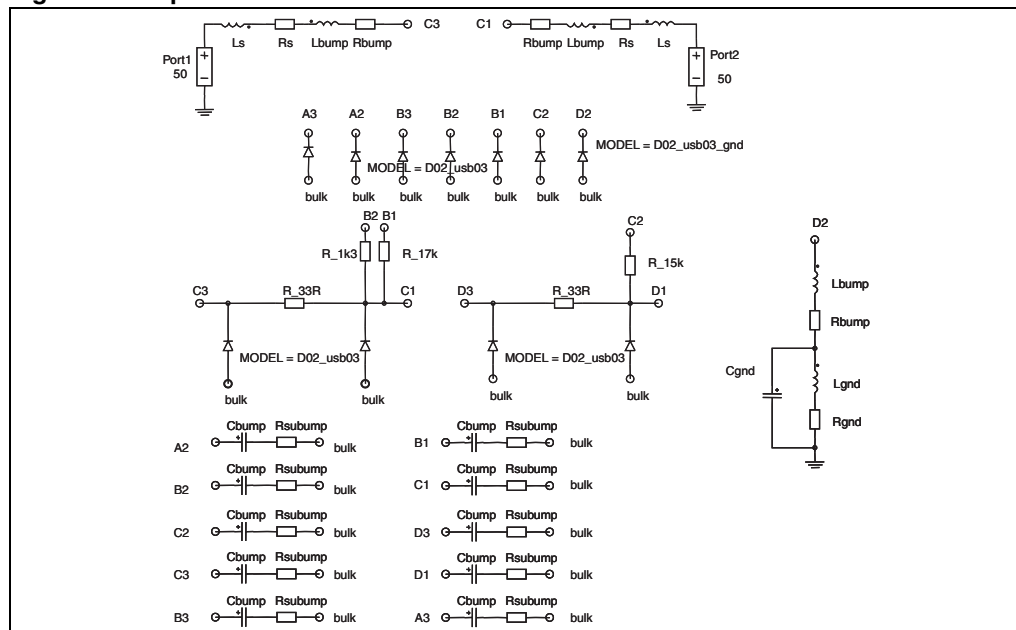
Figure 10. Aplac parameters
