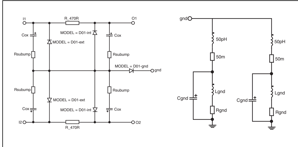
Figure 10. Aplac parameters
