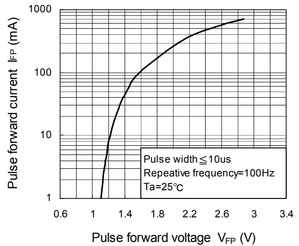
I_{FP} - V_{FP}
