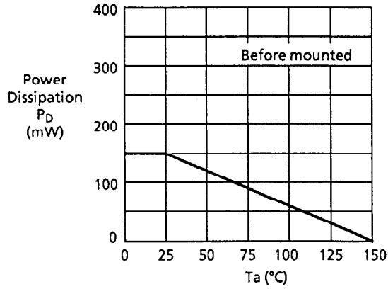
(3) SOT-23-5
