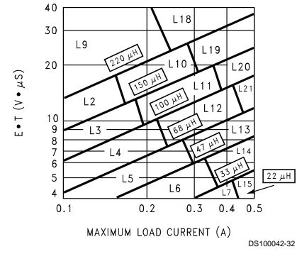
FIGURE 7. LM2671-ADJ
