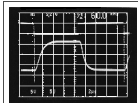
Transmitter Output R_L=3k\Omega , C_L=2,500pF
