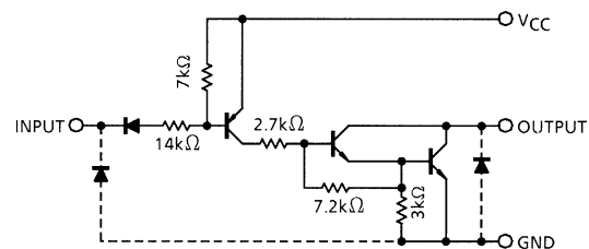
TD62305AP/AF
