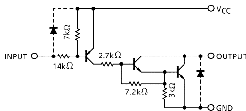
TD62304AP/AF
