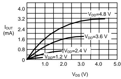
V_{DS} - I_{OUT}
