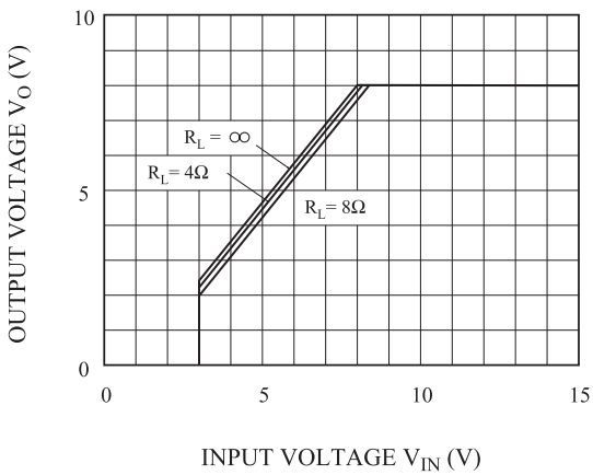
Fig.6-2 V_{IN} - V_O (KIA278R08)
