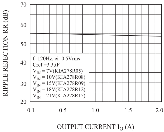
Fig.10-2 I_O - RR
