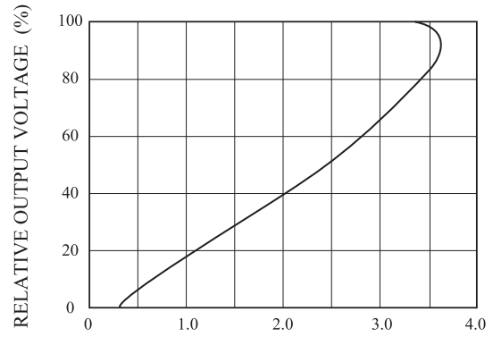
Fig.4 I_O - V_O
