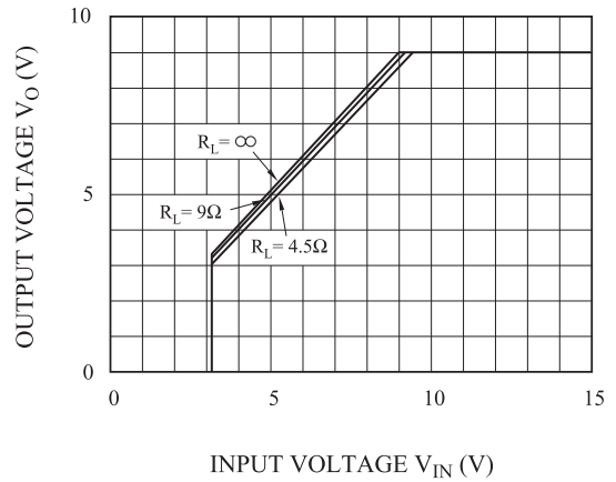
Fig.6-3 V_{IN} - V_O (KIA278R09)
