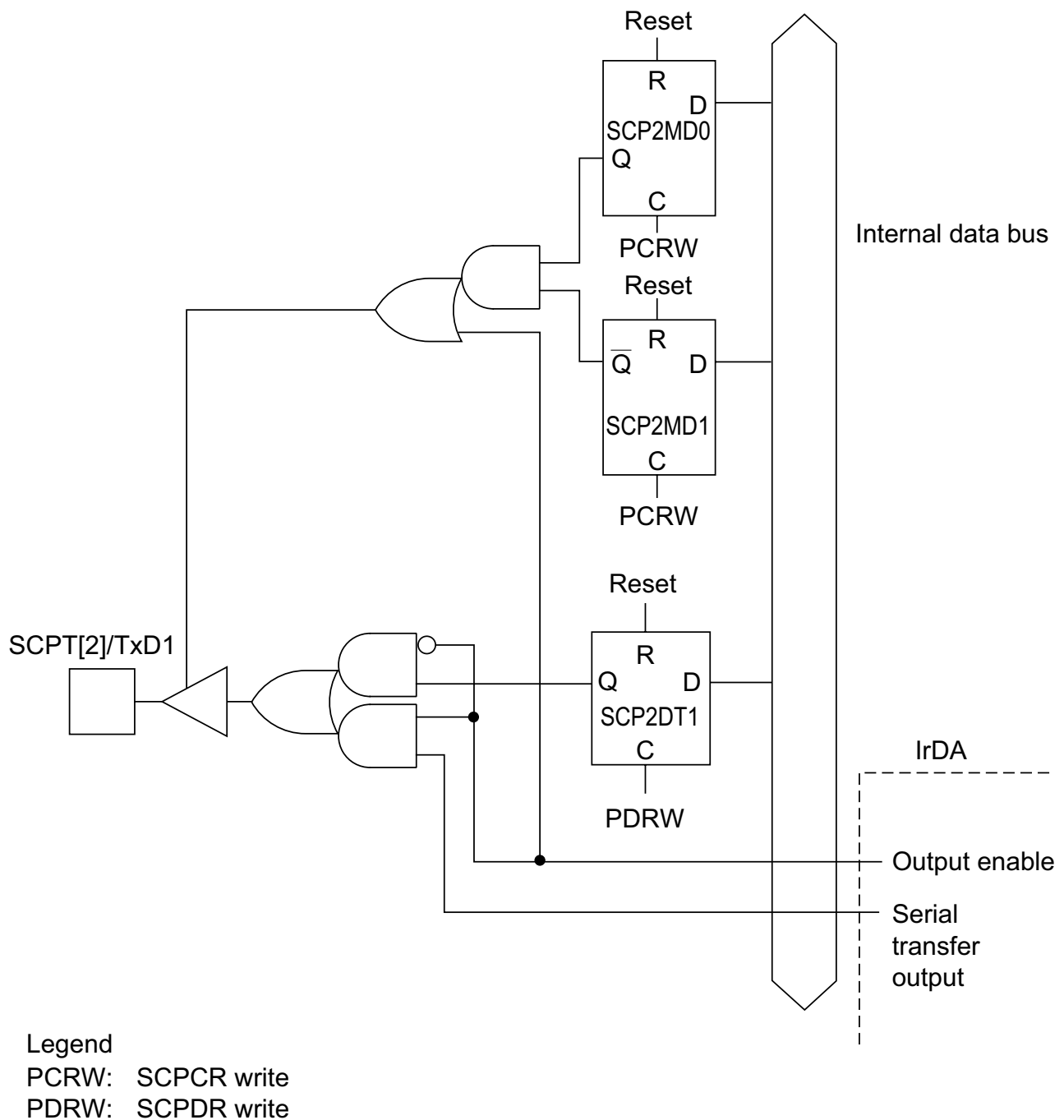
Figure 17.3 SCPT[2]/TxD1 Pin
