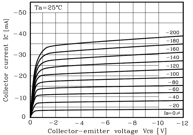
Fig. 2 I_C - V_{CE}
