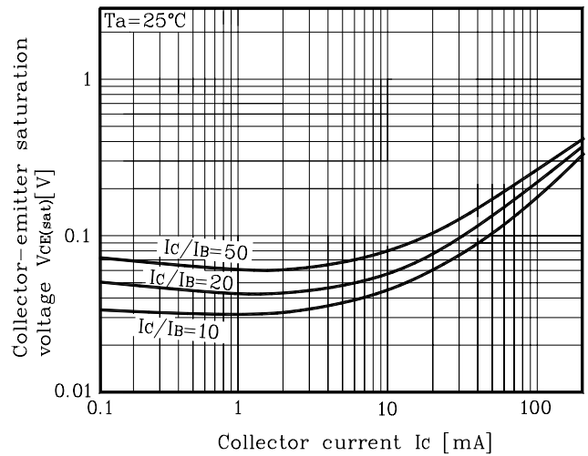
Fig. 2 I_C - V_{CE}
