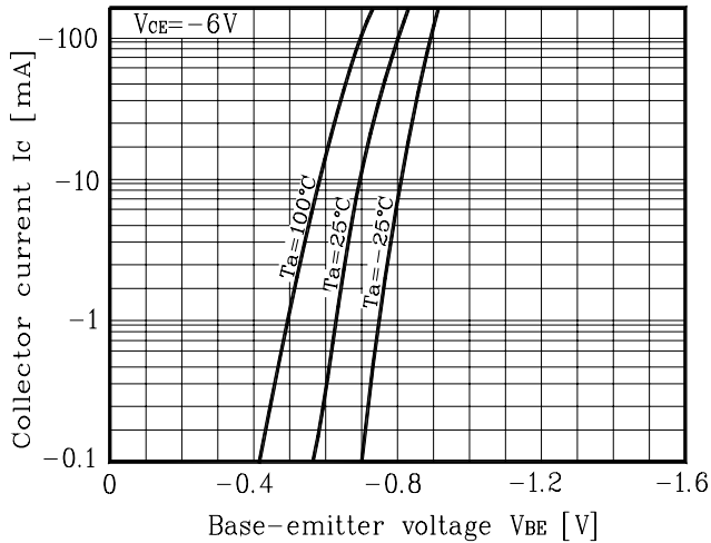
Fig. 1 I_C - V_{BE}
