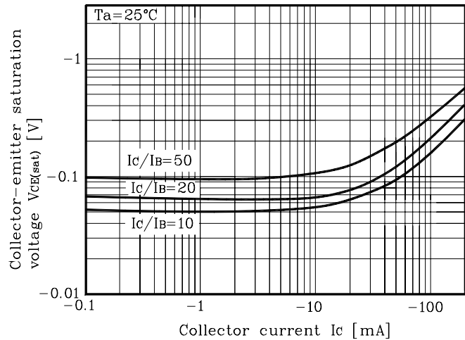
Fig. 4 V_{CE(sat)}-I_C
