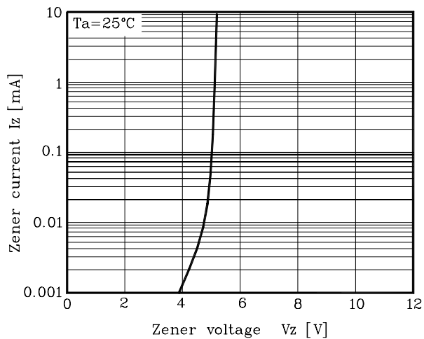
Fig. 2 I_Z - V_Z
