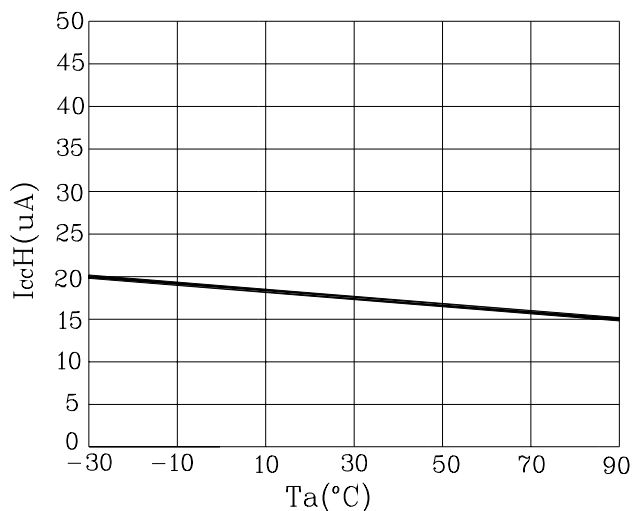
Fig. 3 I_{CCH} - T_a
