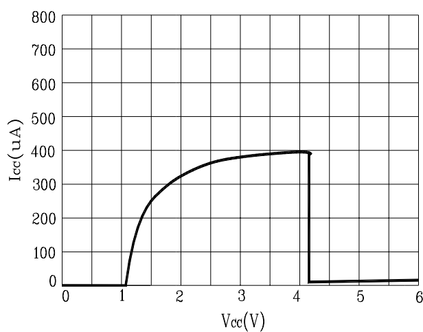
Fig. 2 I_{CC} - V_{CC}
