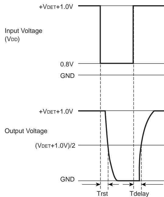
CMOS Output
