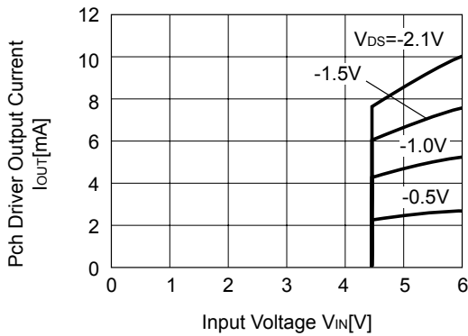
R3130N44xx
