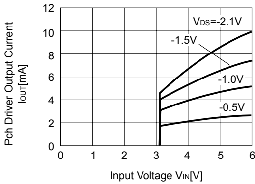
R3130N30xx8
