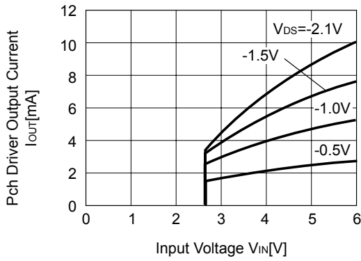
R3130N26xx3
