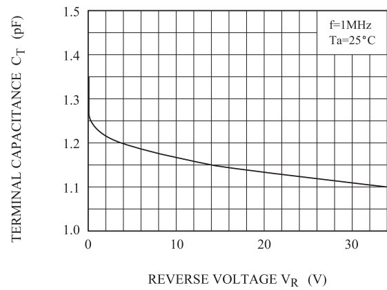
C_T - V_R
