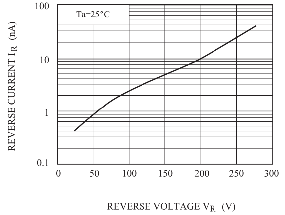
I_R - V_R
