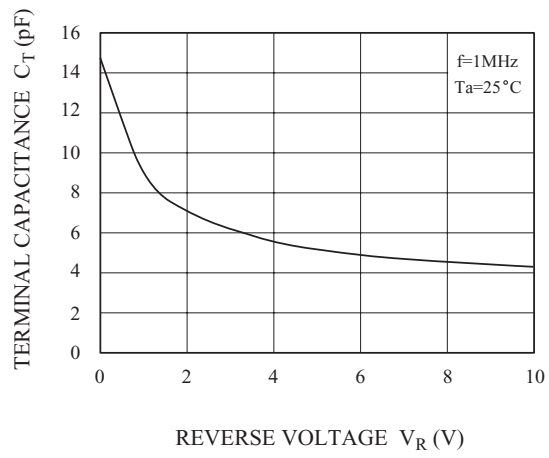
C_T - V_R
