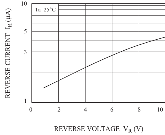
I_R - V_R
