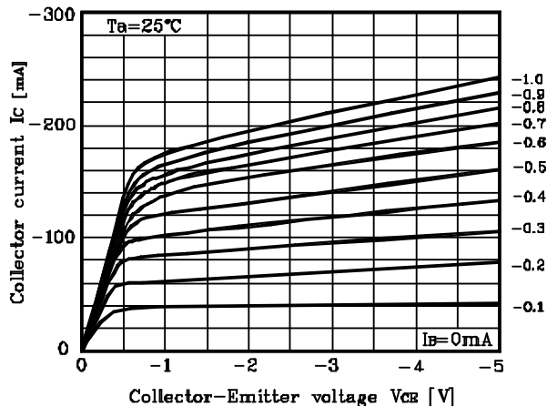
Fig. 4 I_C - V_{CE}
