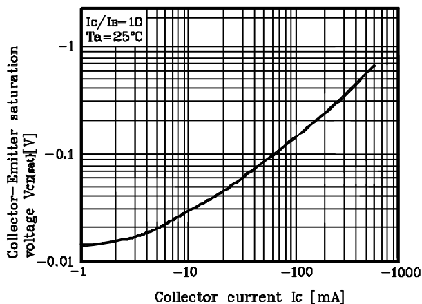
Fig. 5 V_{CE(sat)} - I_C
