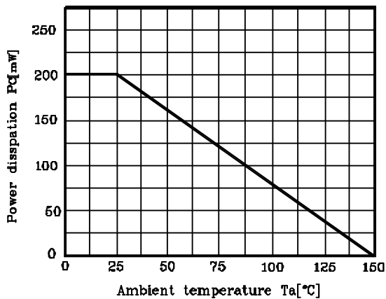
Fig. 1 P_C - T_a
