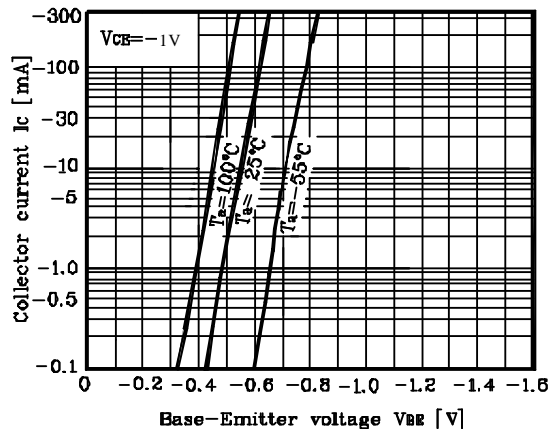
Fig. 2 I_C - V_{BE}
