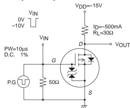
スイッチングタイム測定回路図
