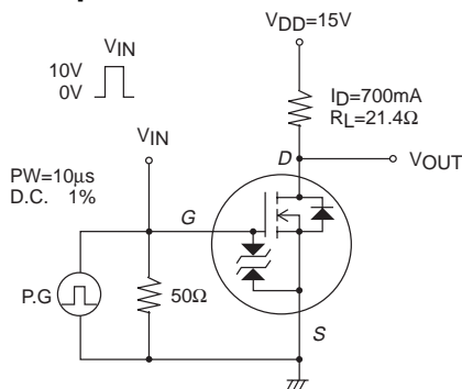
スイッチングタイム測定回路図
