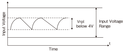
Fig.2-1: Input Ripple Voltage
