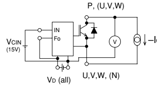
Fig. 2 V_{EC} Test
