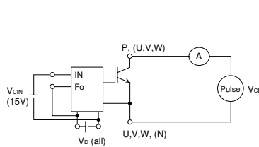
Fig. 5 I_{CES} Test
