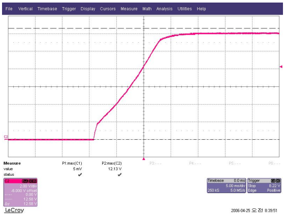
SFS5-12 0V
