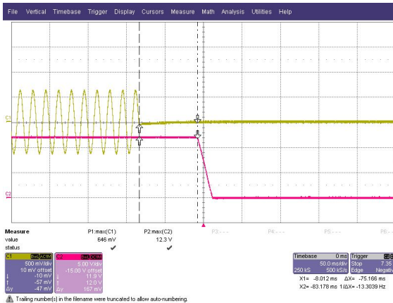
SFS5-12 75ms
