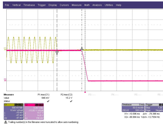
SFS5-15 78ms
