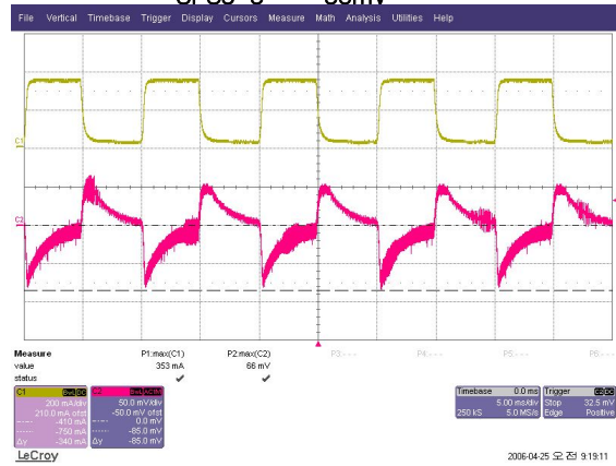
SFS5-15 85mV
