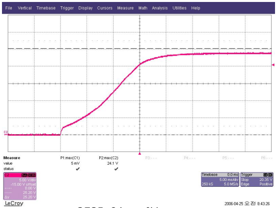
SFS5-24 0V
