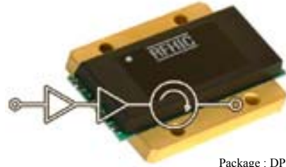
Package : DP-56
