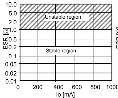
Fig.28 BA3259HFP ESR
