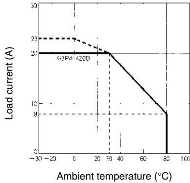
G3PA-420B-VD, G3PA-420B-VD-2
