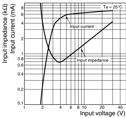
G3PA-2□0B-VD
