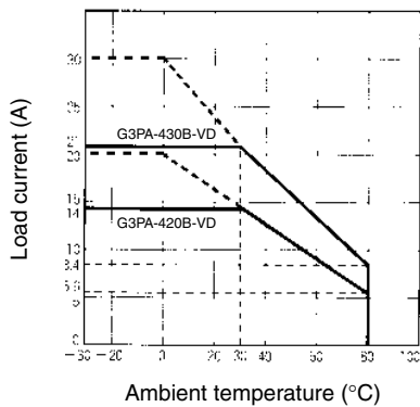
G3PA-420B-VD, G3PA-430B-VD G3PA-420B-VD-2, G3PA-430B-VD-2
