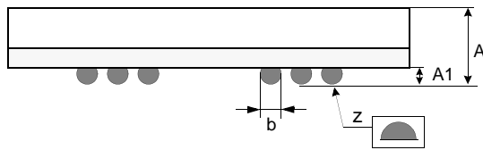
< Top View*2 >
