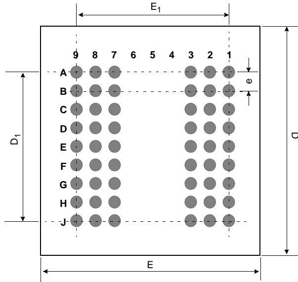
< Bottom View*1 >
