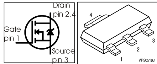
SOT-223
