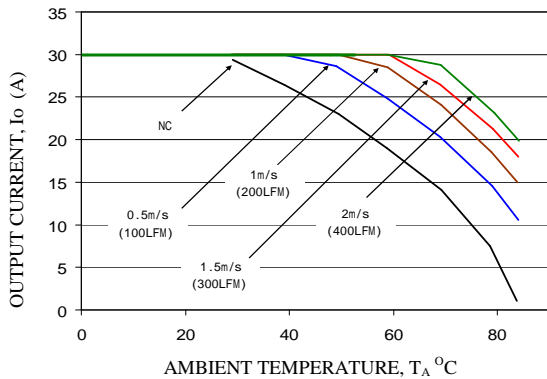
Vo=3.3V, Vin=12V
