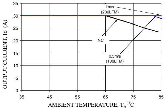
Vo=0.8V, Vin=12V
