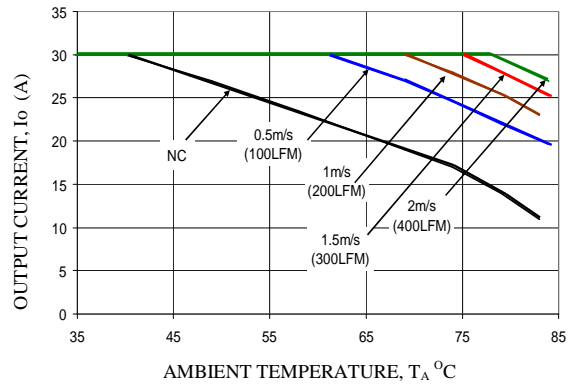
Vo=2.5V, Vin=12V
