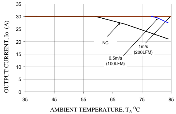
Vo=1.2V, Vin=12V
