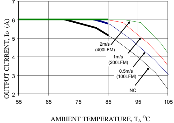
V_o=5.0V
