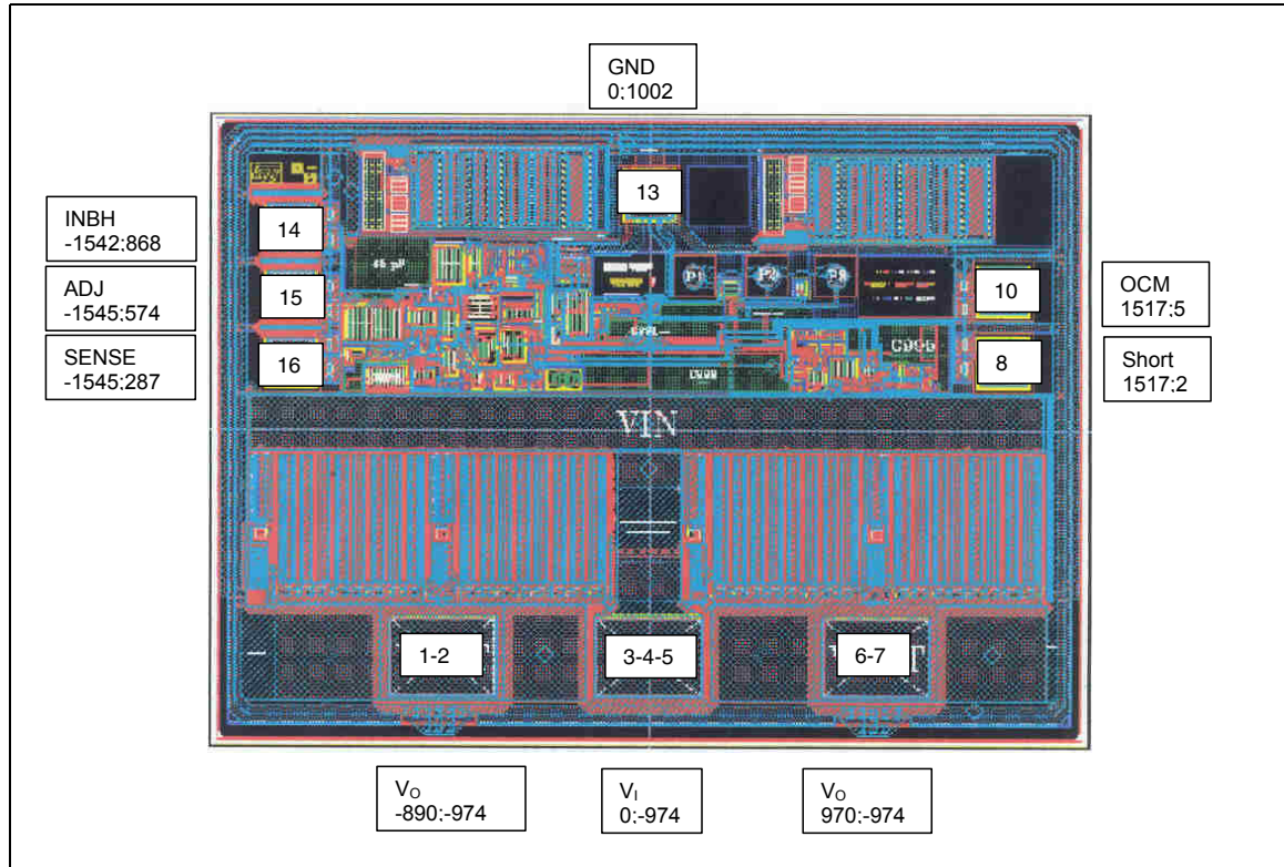
Figure 4. Die map
