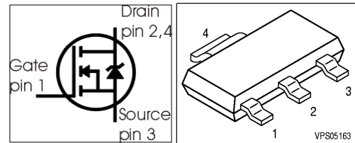
PG-SOT223
