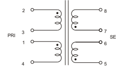
2. SCHEMATIC :
