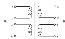
2. SCHEMATIC :
