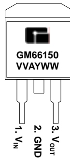
TO 263 (D 2 -PAK)
