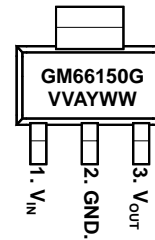
SOT223
