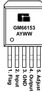
TO-263-5
