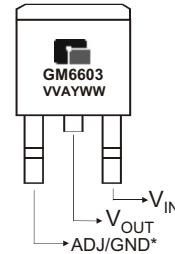
TO-263-2 (D 2 PAK)
